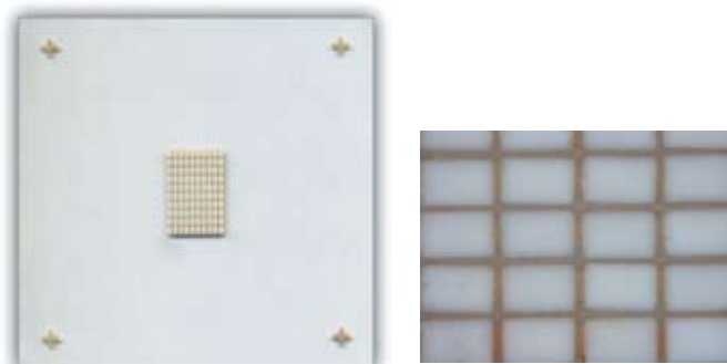
Рис. 2 Тестовый образец для определения качества отмытки и эффективности работы оборудования
