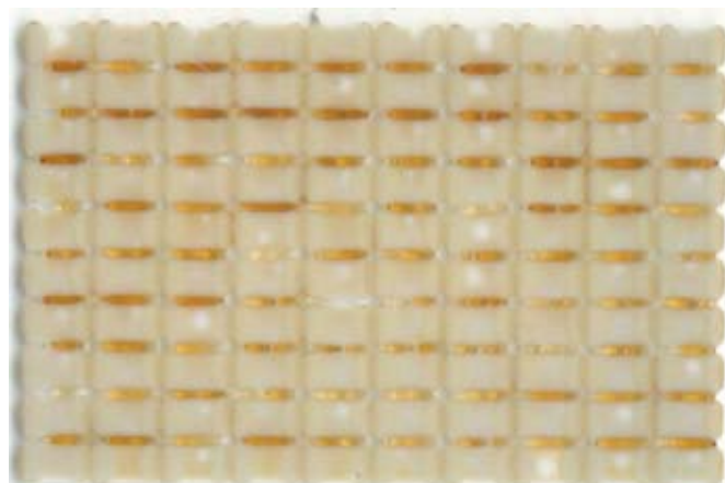
Рис. 13 Результаты эксперимента с применением барботажа. Наличие остатков флюса видно невооруженным глазом
