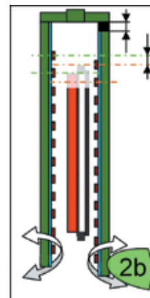
Рис. 10 Схема процесса отмывки с форсунками, плавно и поступательно перемещающимися в плоскостях, параллельных отмываемым изделиям
