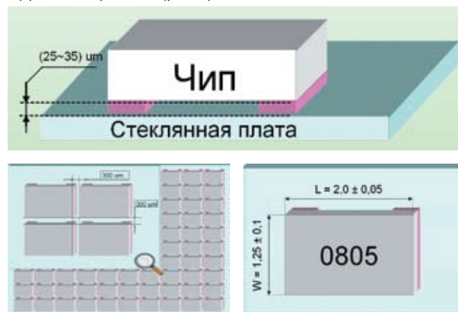
Рис. 1 Описание технологии изготовления тестового образца
