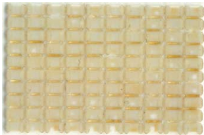
Рис. 12 Результаты эксперимента по технологии «струи в объеме». Очевидны остатки флюса как между, так и под чипами
