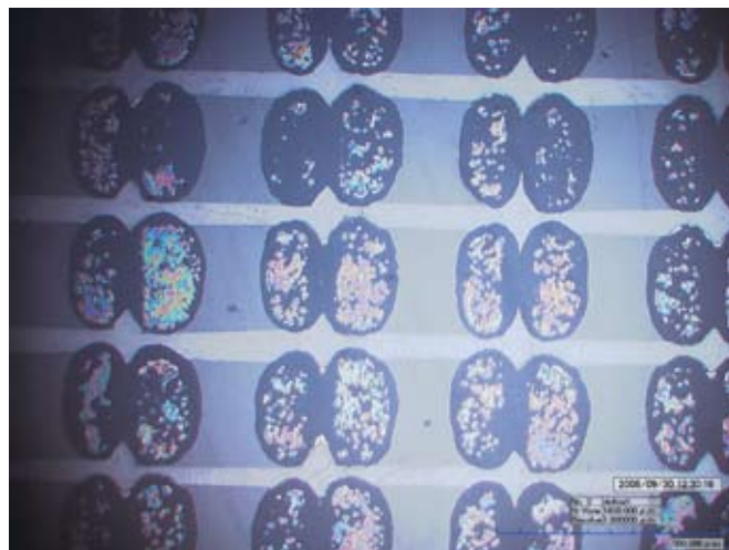
Рис. 4 Изображение отмытой в ультразвуковой ванне платы, полученное на видеомикроскопе Hirox KH-7700
